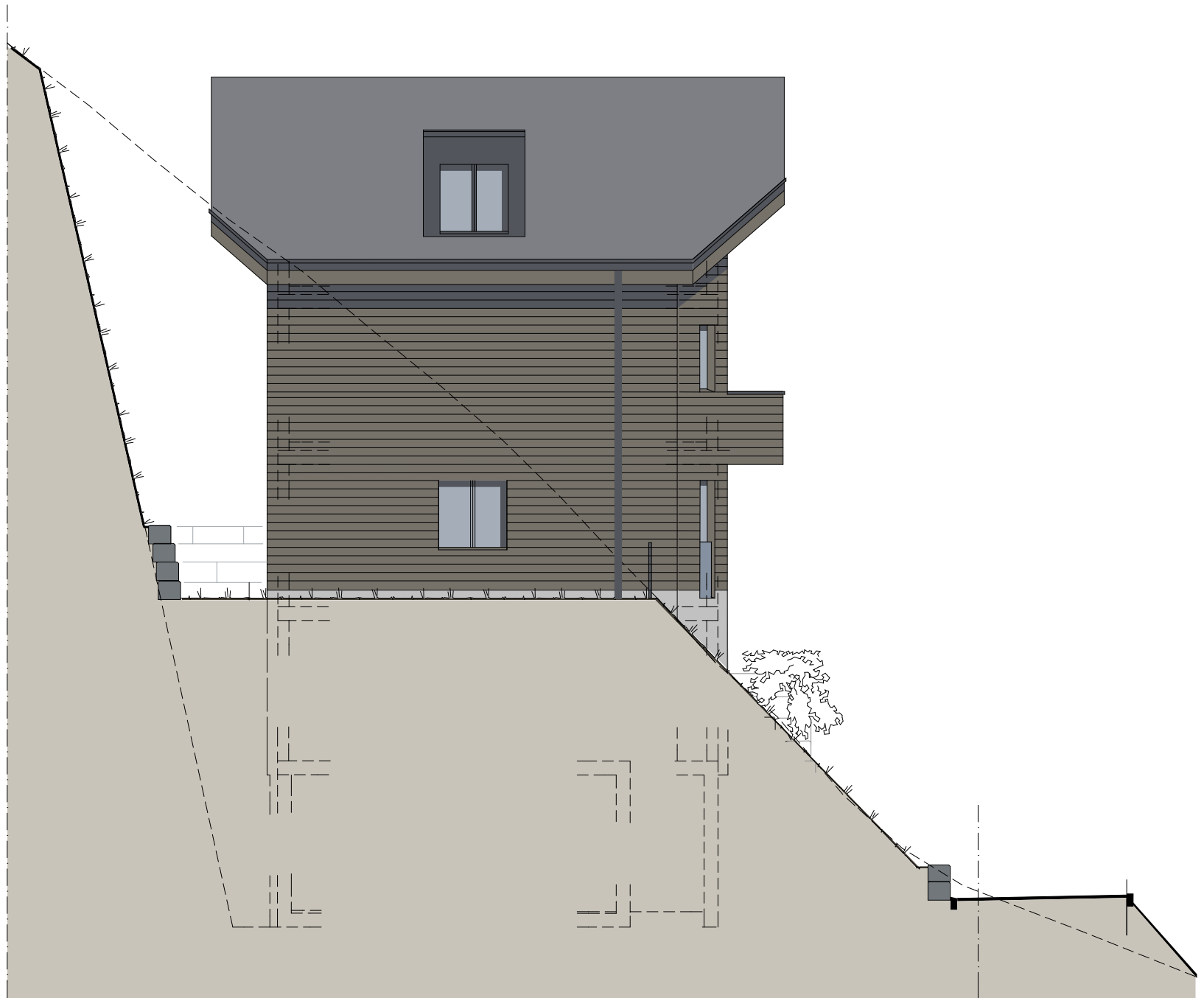
Ansicht West
