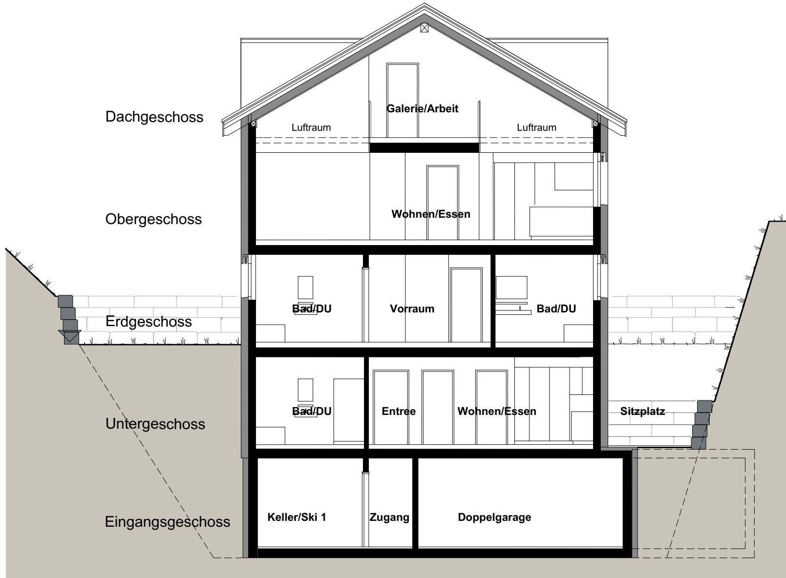
Querschnitt
